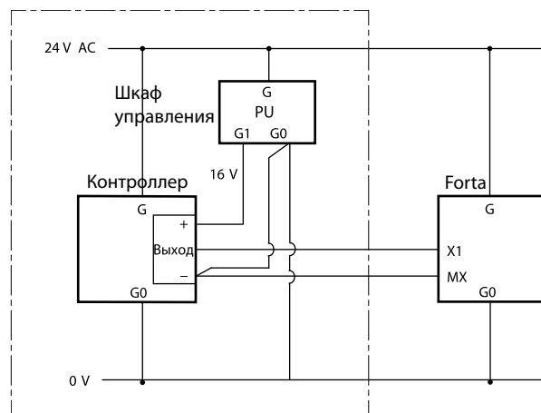
Аналоговое управление, выход контроллера с гальванической развязкой (TAC 6501, TAC 6505)
