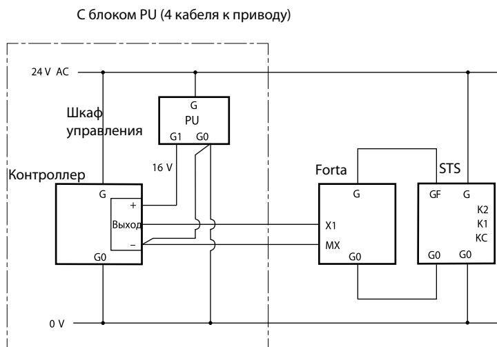
Аналоговое управление, выход контроллера с гальванической развязкой (TAC 6501, TAC 6505)
