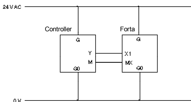
Станд. схема (4 кабеля к приводу)
