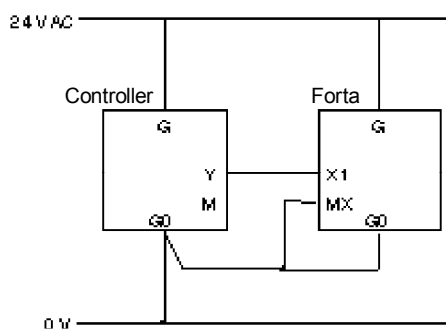
Упрощ. схема (3 кабеля к приводу)
