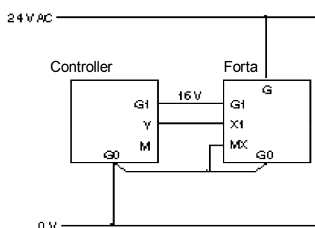
Упрощ. схема (4 кабеля к приводу)
