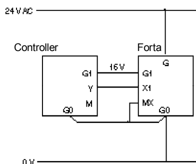
Станд. схема (5 кабелей к приводу)
