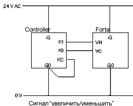
Упрощ. схема (3 кабеля к приводу)
