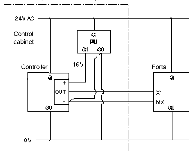
С блоком PU (4 кабеля к приводу)
